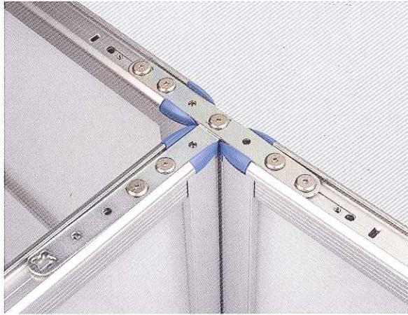
T-connection
